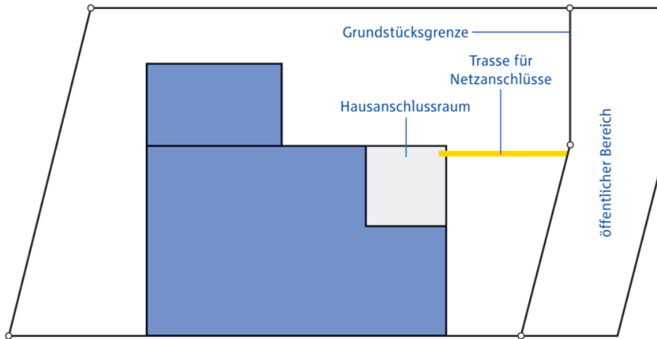
Lageplan für Hausanschlussraum (Beispiel)
